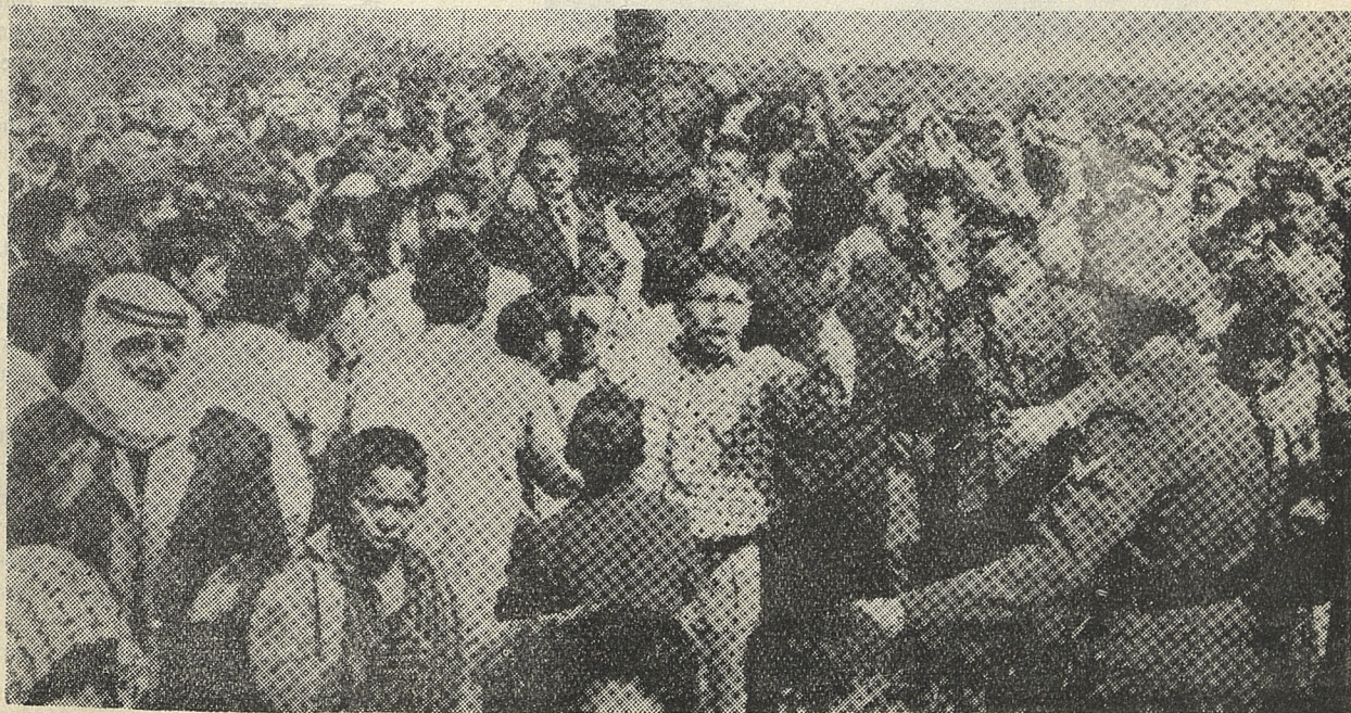
Pueblo sirio expresa su júbilo al distribuirse las tierras, 1.118 familias recibieron 147,000 dunums.
